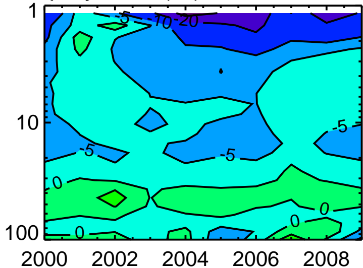
Replay-Obs (%) HauteProvence
