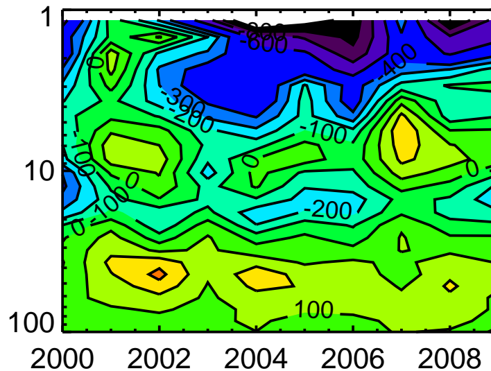
GMI CTM-Obs HauteProvence
