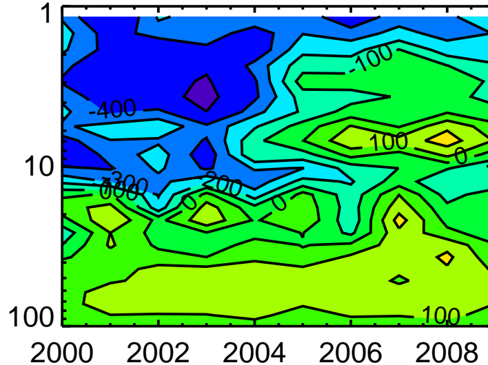
GMI CTM-Obs MaunaLoa
