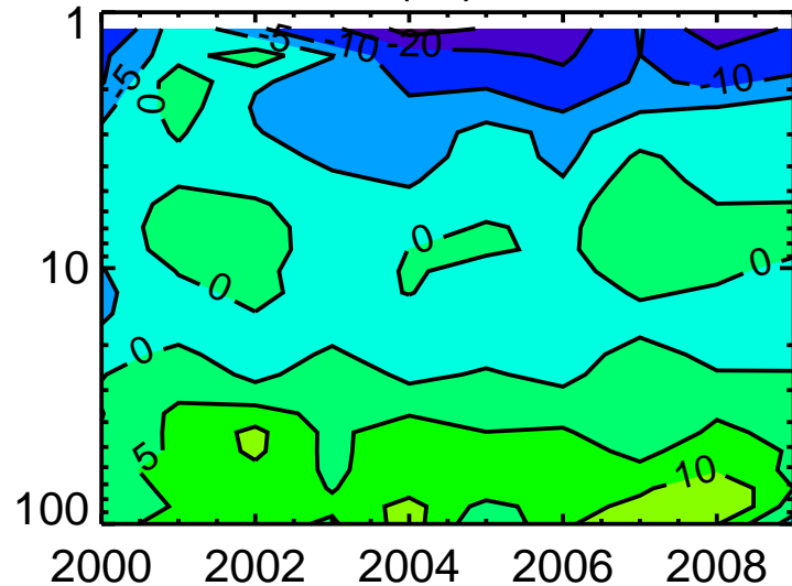
GMI CTM-Obs (%) HauteProvence
