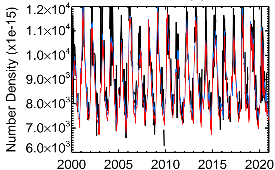
Kiruna O 3
