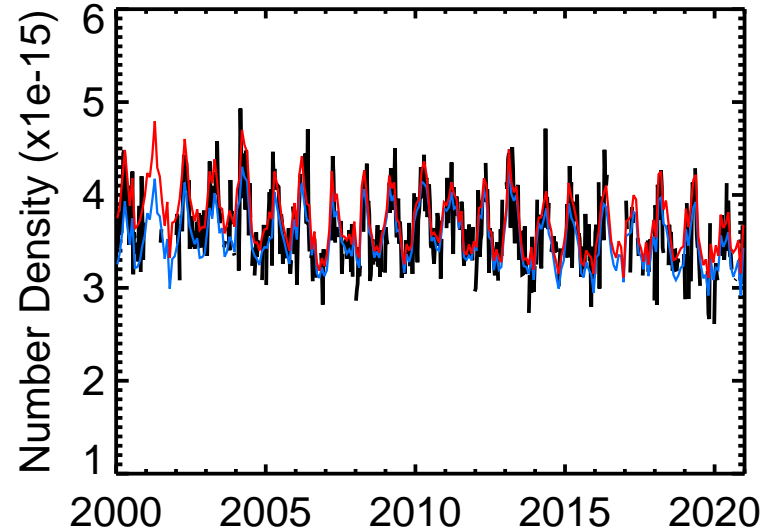
Jungfrau HCl
