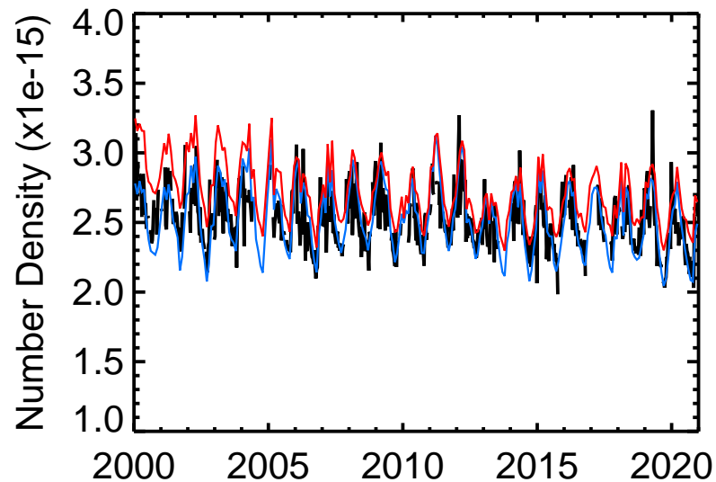
Izana HCl
