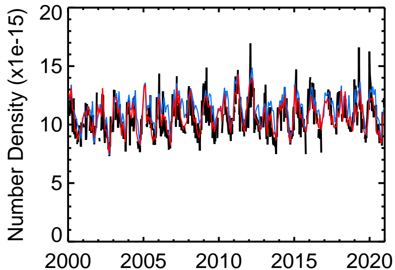
Izana HNO 3
