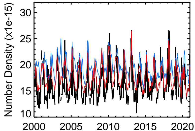
Jungfrau HNO 3
