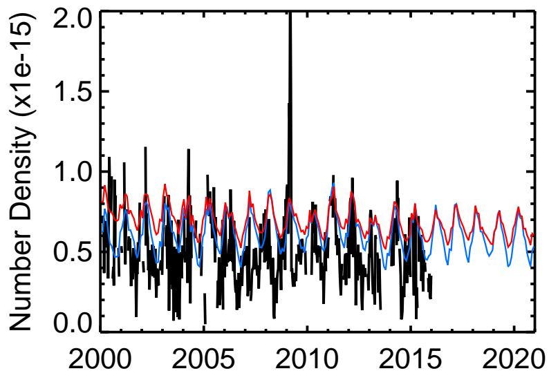
Izana ClONO 2
