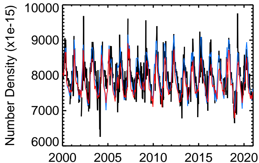
Izana O 3
