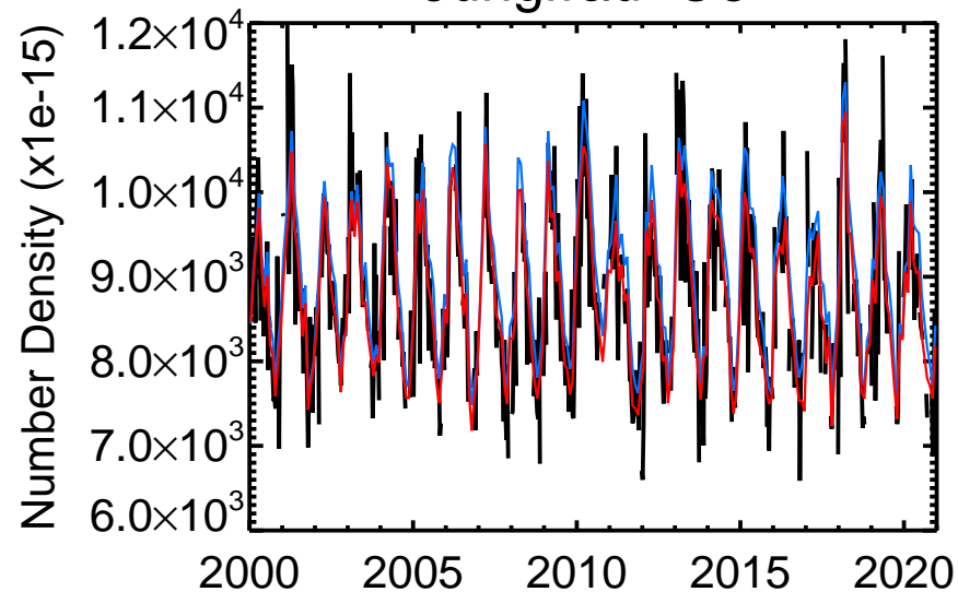
Jungfrau O 3
