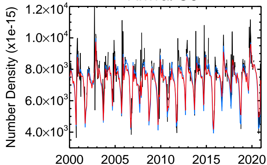
Arrival O3
