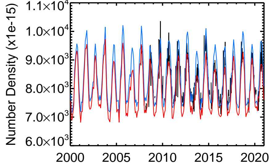
Wollongong O 3
