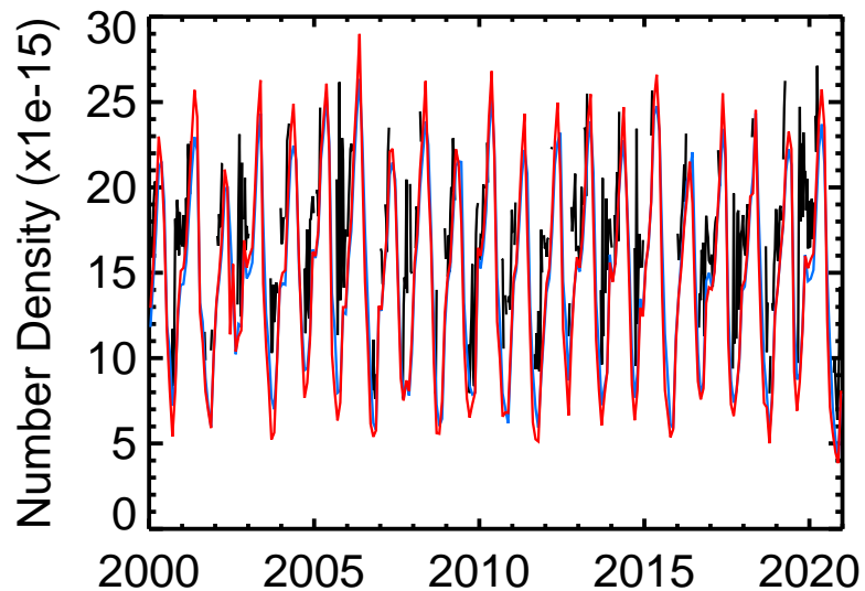
Arrival HNO3
