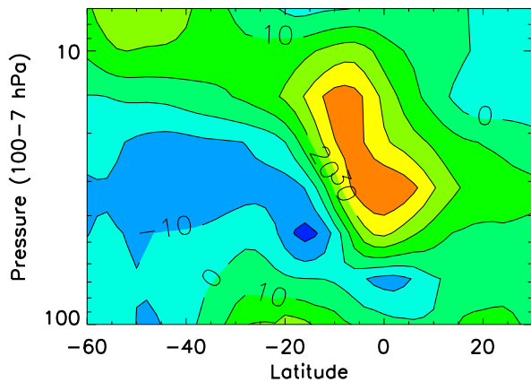
2022 HNO 3 Anom SEP
