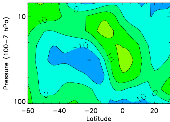
2015 HNO 3 Anom SEP
