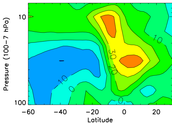
2022 HNO 3 Anom OCT
