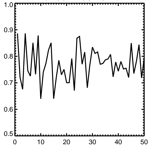
10-18S HNO3 4.6 mb
