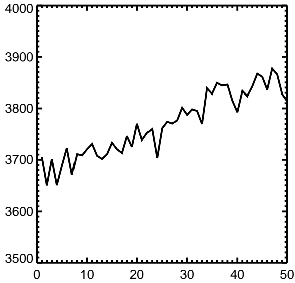
10-18S O 3 31 mb
