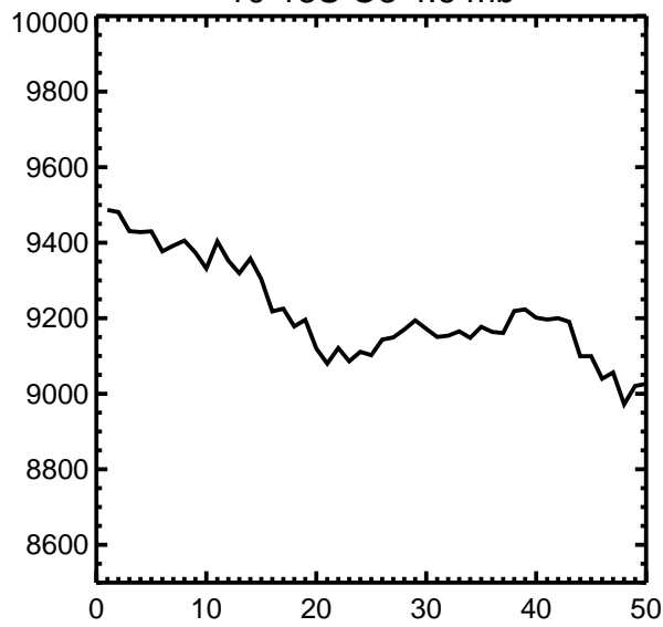
10-18S O3 4.6 mb
