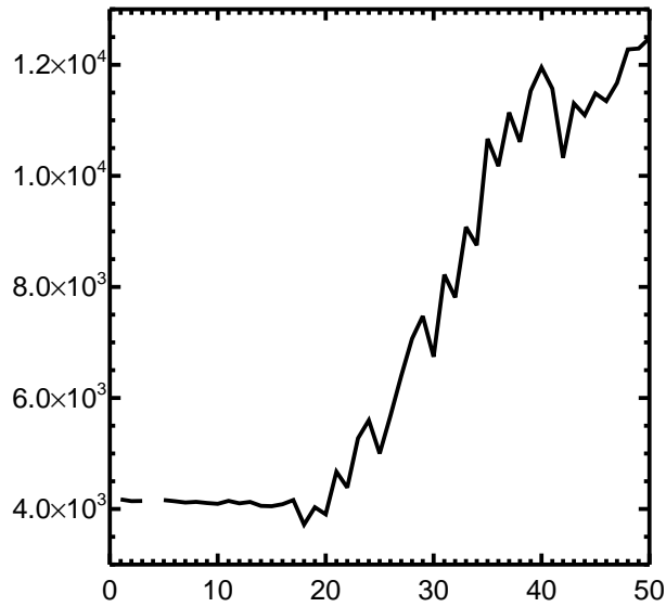
10-18S H 2 O 31 mb
